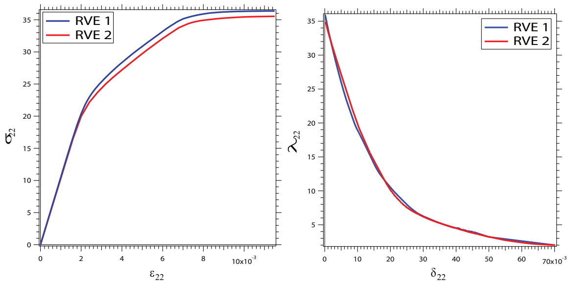
(a) Curva Tensión-deformación previo a la pérdida de (b) Curva Tensión-Salto posterior a la pérdida de elip- ticidad. Modelo Clásico. ticidad. Modelo Propuesto.
