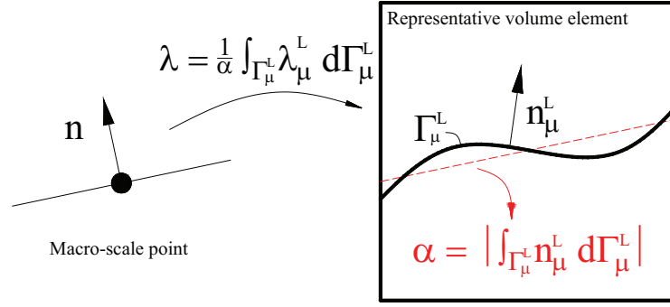
Figura 3: Esquema de la cinemática de la transición de escala.
