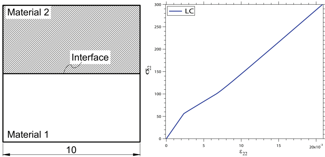
(a) RVE con fisura atravesando el borde. (b) Gráfico \sigma versus \varepsilon para condición de borde LC.
